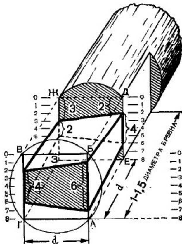
Р и с. 89. Рубка углов стен «в лапу» и порядок ее разметки
